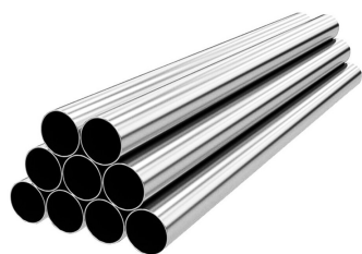
VZWSMART 150" PIPE 2.5 SCH40 (2.875" OD X 0.203" THK)
